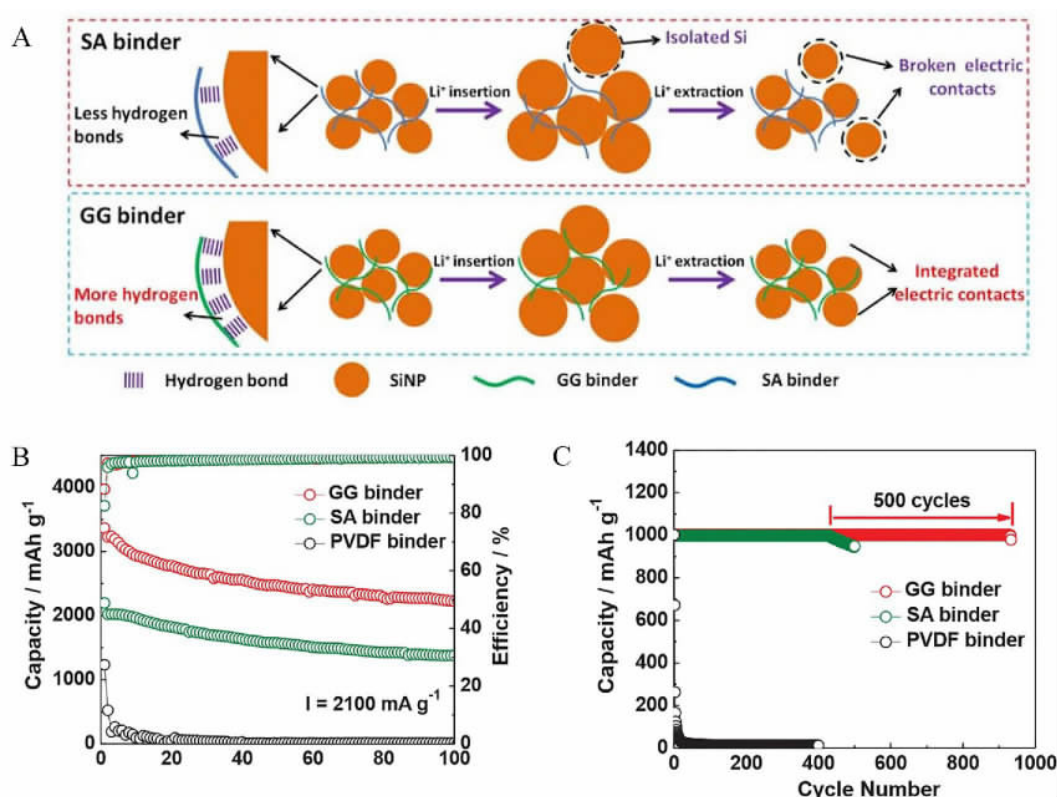
图 4 (A) 海藻酸钠与瓜尔豆胶构建的导电网络在充放电过程中变化的示意图; (B) 不同粘结剂在 0.01 \sim 1.2 \text{ V} , 2100 \text{ mA} \cdot \text{g}^{-1} 条件下充放的循环性能比较; (C) 不同粘结剂在 1000 \text{ mA} \cdot \text{g}^{-1} 条件下限制 1000 \text{ mAh} \cdot \text{g}^{-1} 容量充放的循环性能比较 [45]
