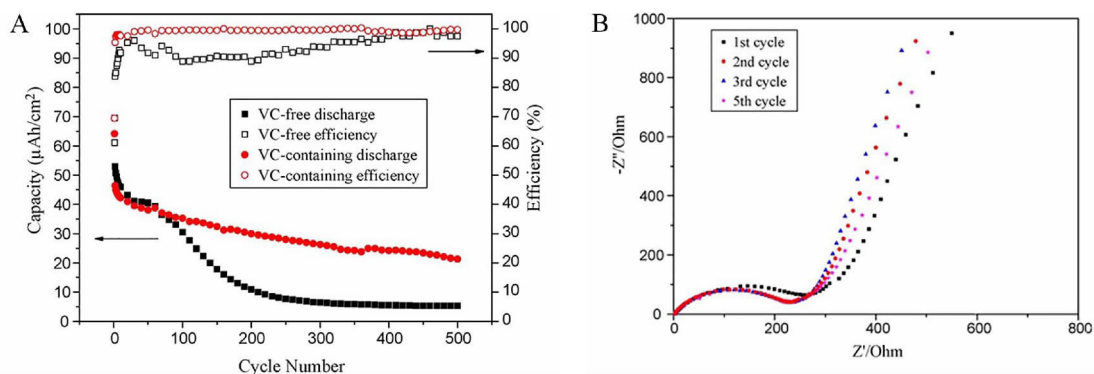
图 7 (A) VC 添加剂对硅薄膜电极循环性能的影响; (B) 加入 VC 添加剂的硅薄膜电极的阻抗分析 [58]
