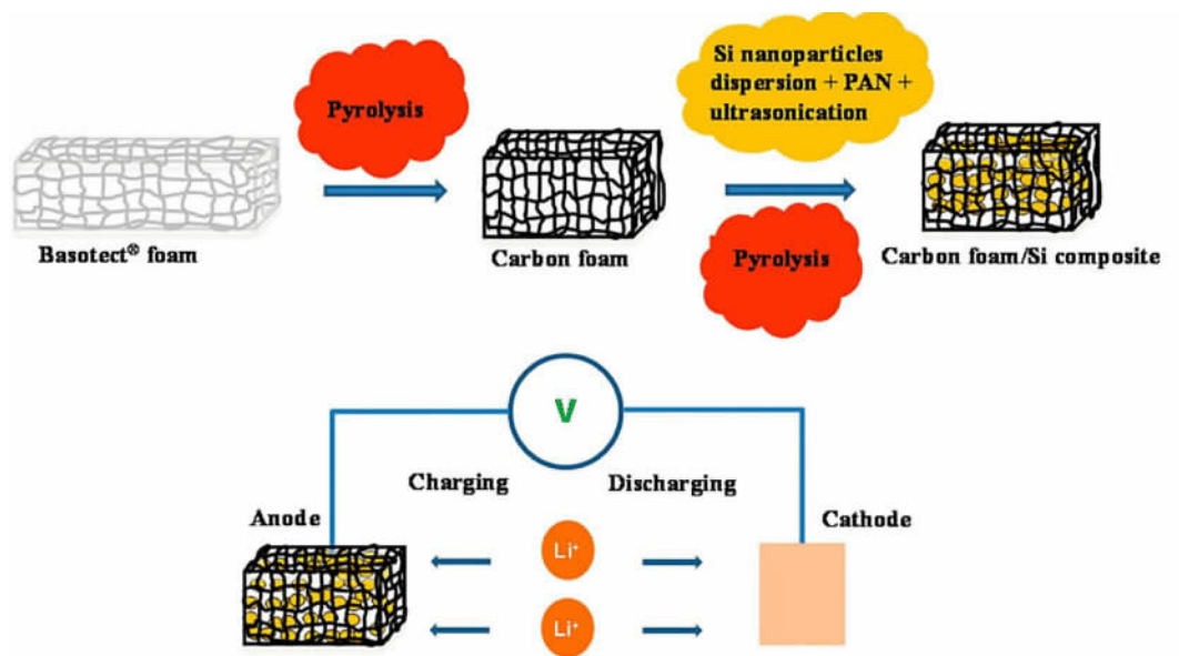
图 6 制备泡沫碳/硅复合电极的主要示意图 [52]
