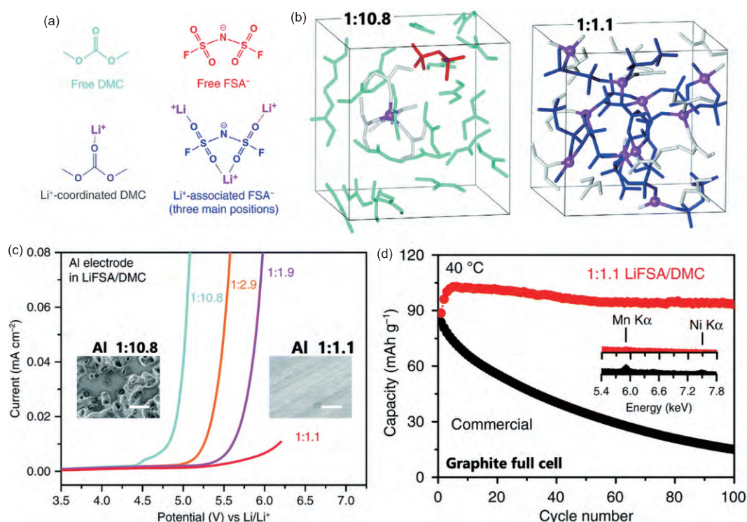
图3 具有良好电化学稳定性的用于高电压 \text{LiNi}_{0.5}\text{Mn}_{1.5}\text{O}_4 材料的LiFSA/DMC电解液体系. (a) LiFSA/DMC混合电解液中的组分结构示意图; (b) 两种不同配比情况下, 溶剂分子典型平衡轨迹的DFT-MD模拟; (c) 铝电极在LiFSA/DMC混合电解液中的高电压稳定性; (d) 全电池在40°C, C/5倍率下的循环性能 [31] (网络版彩图)
